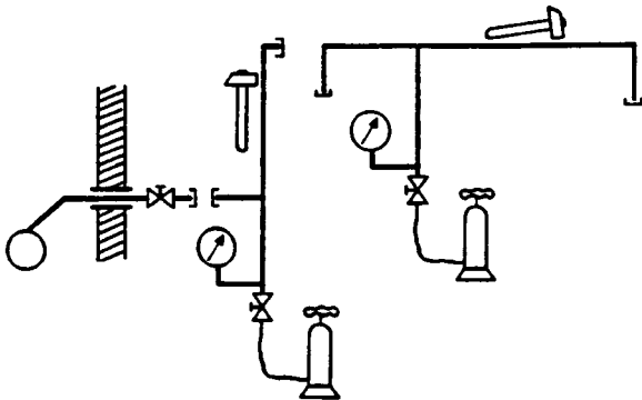
Εικόνα 12.1 Δοκιμή αντοχής
