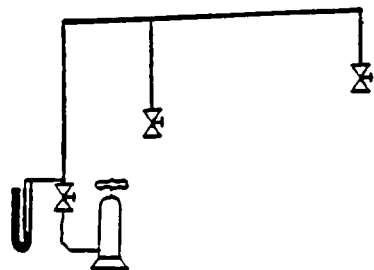
Εικόνα 12.2 Δοκιμή στεγανότητας
