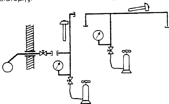
Εικόνα 10.1 Δοκιμή αντοχής
